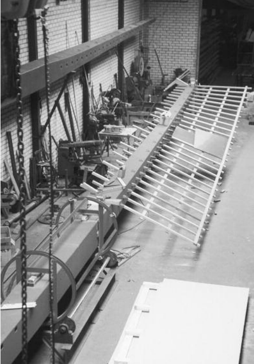
De roeden voor de molen van Silvolde in de maak in de werkplaats van molenmaker Vaags in Aalten (foto A. Nibelink, 11 juli 1999).
