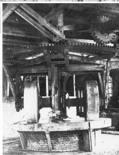
Kollergang van een loodwitmolen met op de achtergrond karren met lappen lood. Deze stond tot circa 1945 in een loodwitfabriek in Schoonhoven en werd oorspronkelijk door een paard gedreven.
