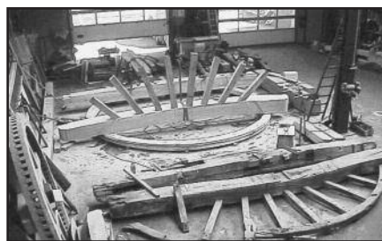
De nieuwe kap voor de Sevink Mølle in aanbouw in de werkplaats van molenmaker Vaags (foto A. Nibbelink)
