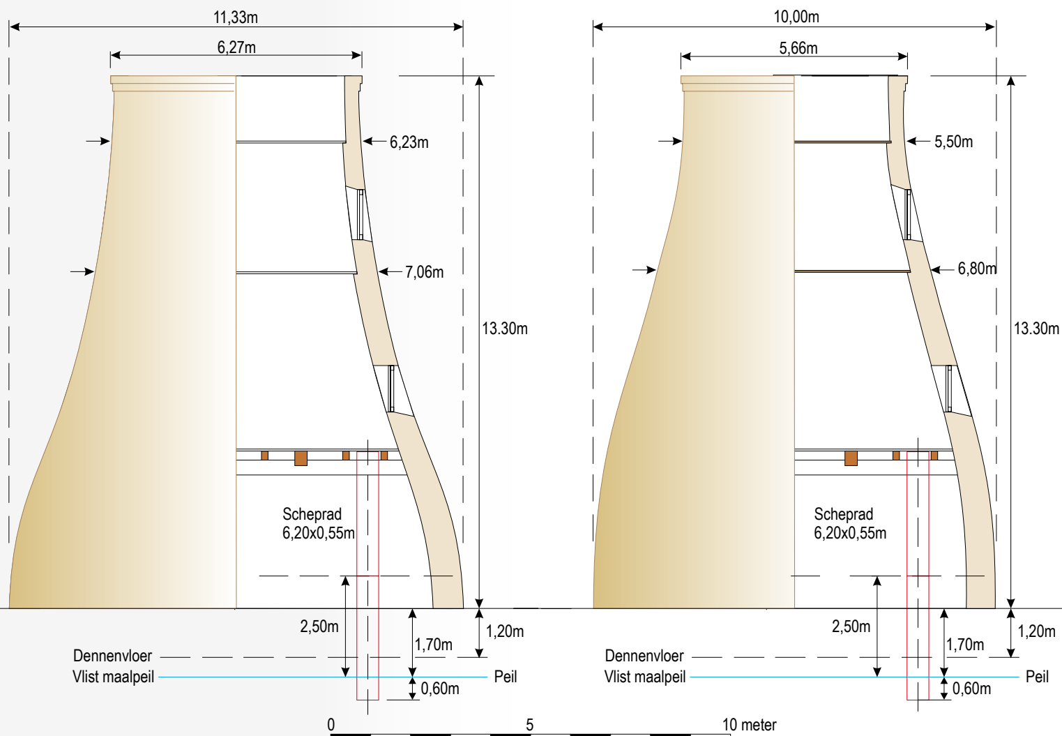
▲ De Haastrechtse molen 6: links de bestaande romp en rechts zoals hij volgens het bestek uit 1873 zou moeten worden (tekening Bas Koster).
