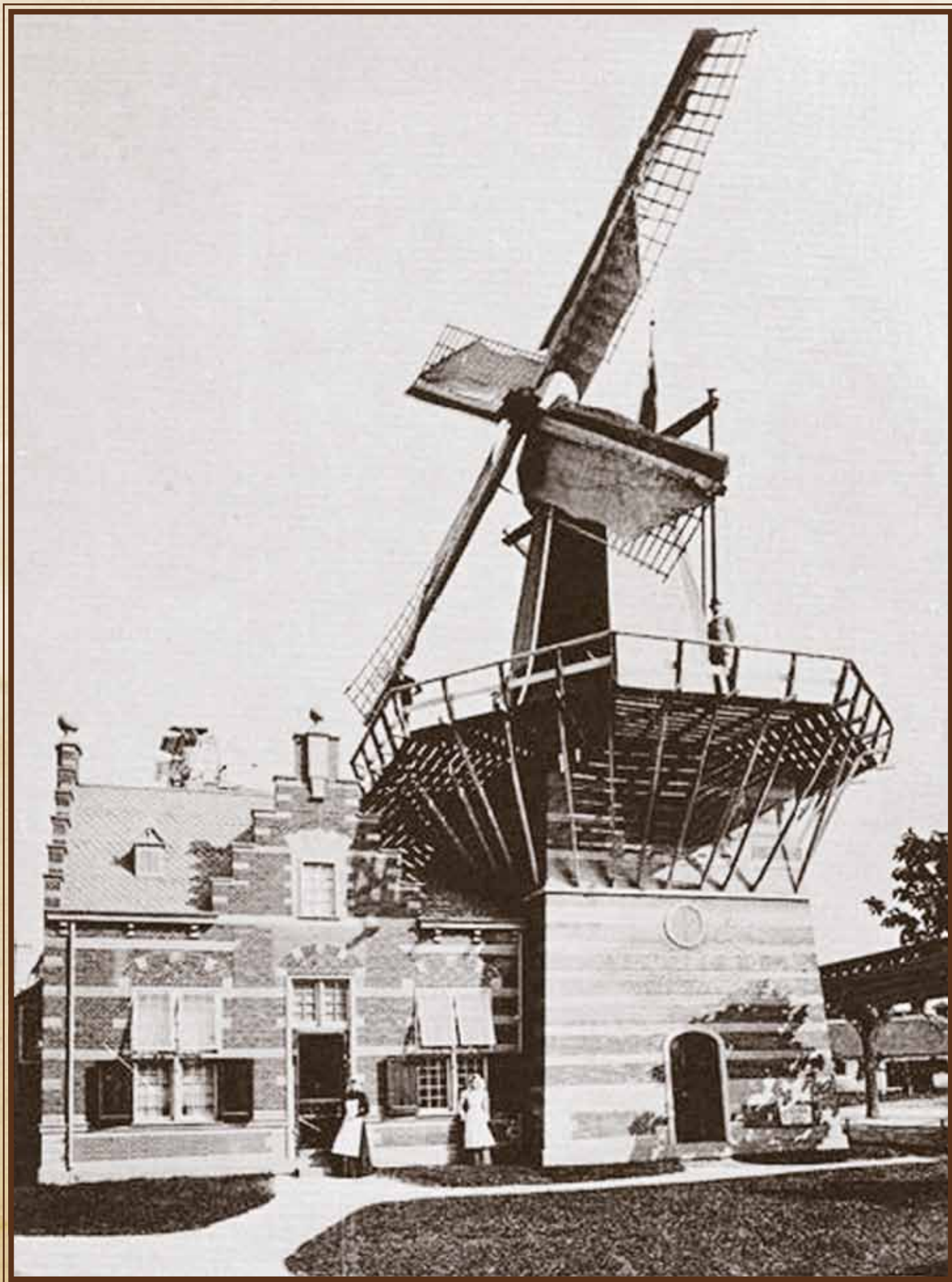
▲De molen van Bloeker op de werldeftoonftelling in Chicago in optima forma. De balie is iel uitgevallen. Het achtkant is veel te strak en glad voor het mooi, maar de kap en het wiekenkruis maken een volledig authentieke indruk; van de Amsterdamse Bloekermolen? Achter het pand met de trapgevels is nog een windmotor zichtbaar.
